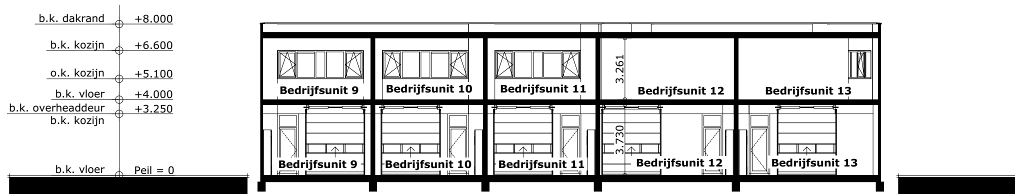
DOORSNEDE B-B
